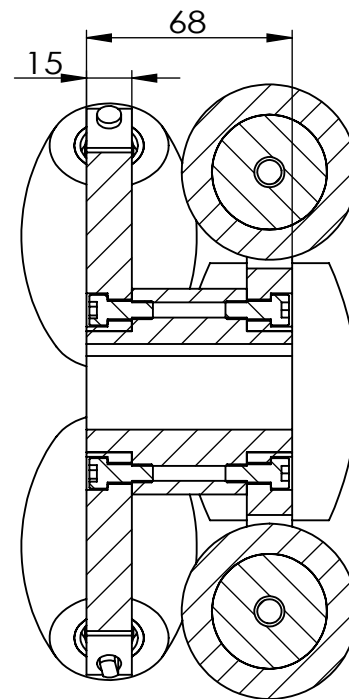
A-A 比例 1 : 2.5
