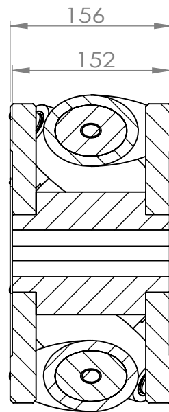
A-A 比例 1 : 5
