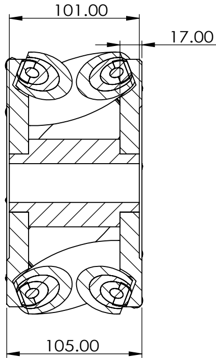
B-B 比例 1 : 3
